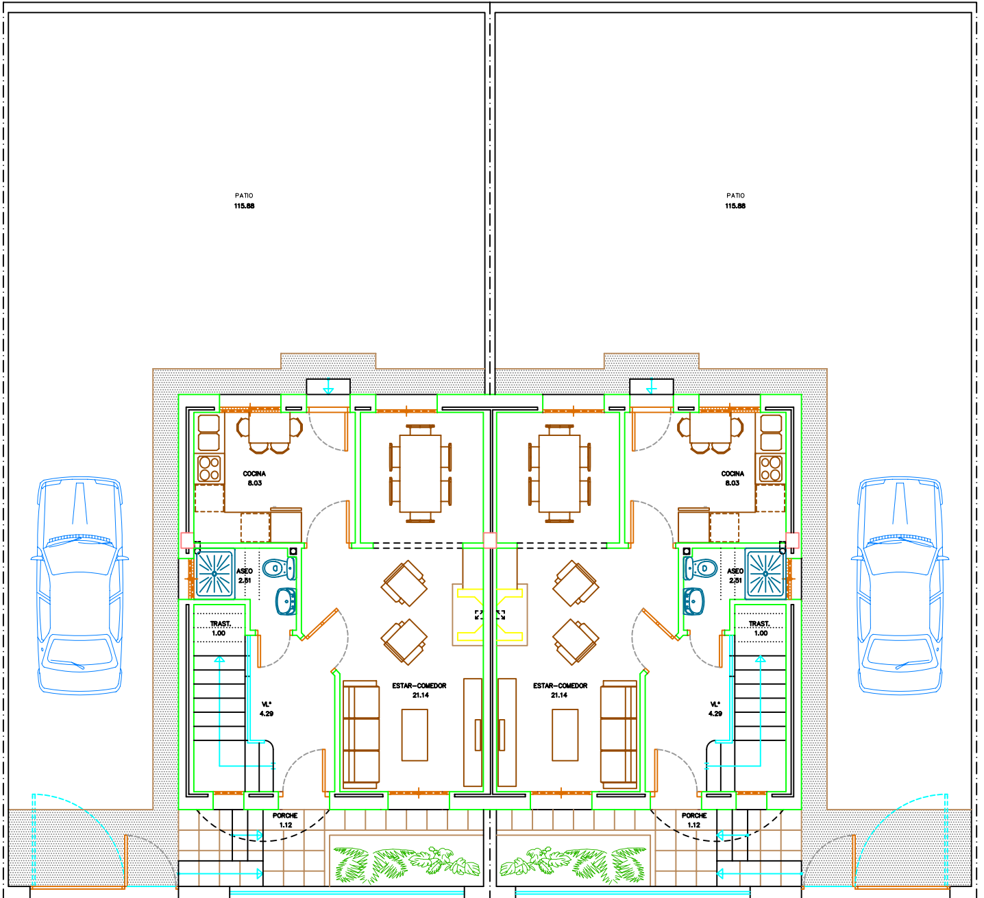
PLANTA BAJA
